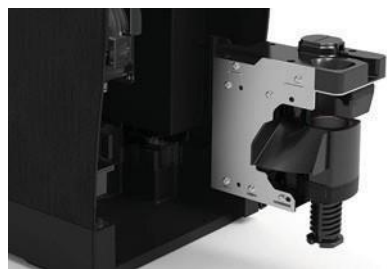
Съемное заварочное устройство с дозировкой до 14 (20) гр., с функцией предсмачивания
